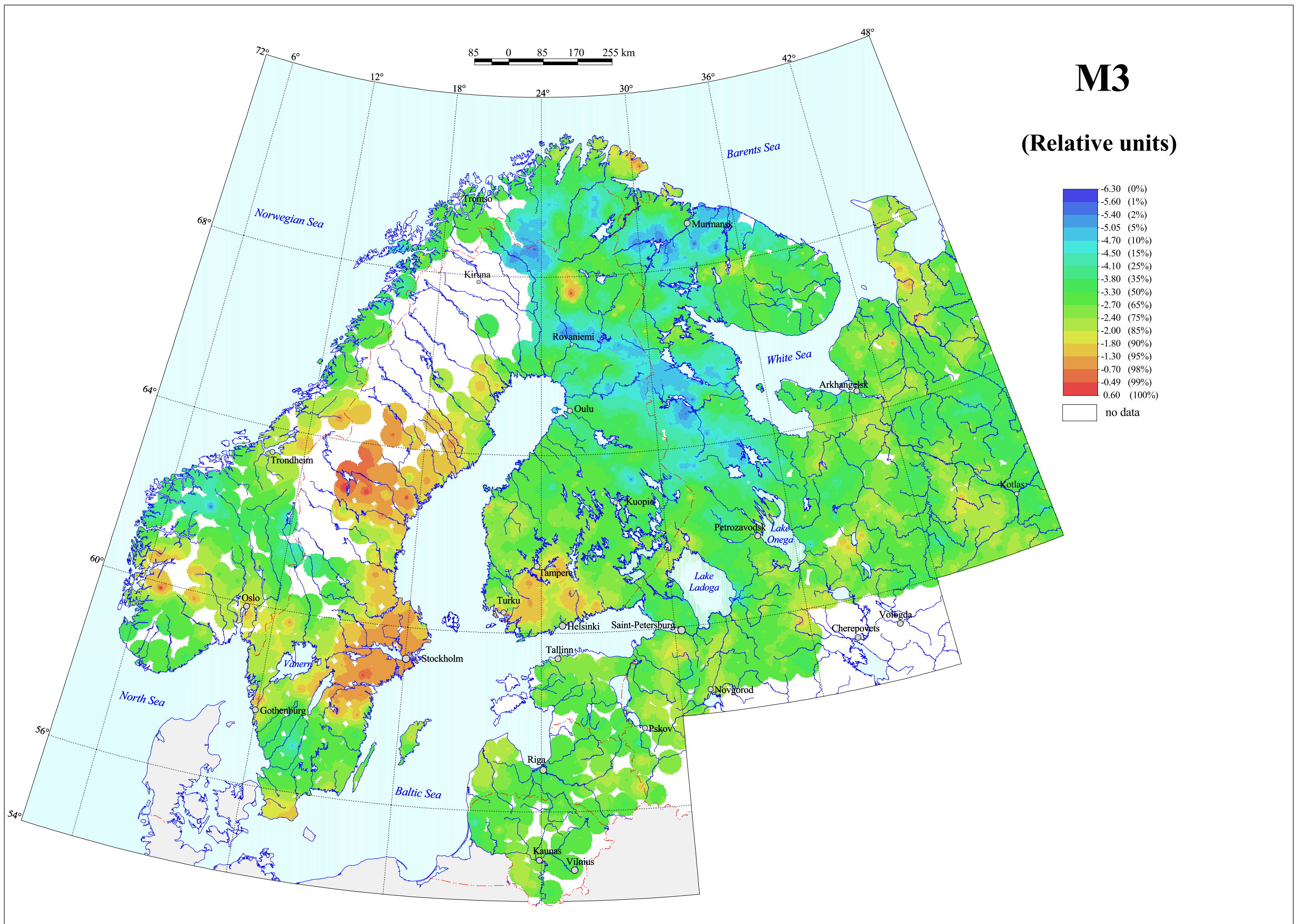
M3 (As, Bi, Cd, Sb, Mo) in C-horizon, Grain Size <2 mm, Aqua regia Extraction
